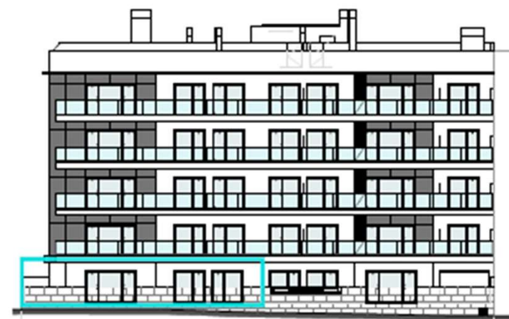
Alçado Poente
