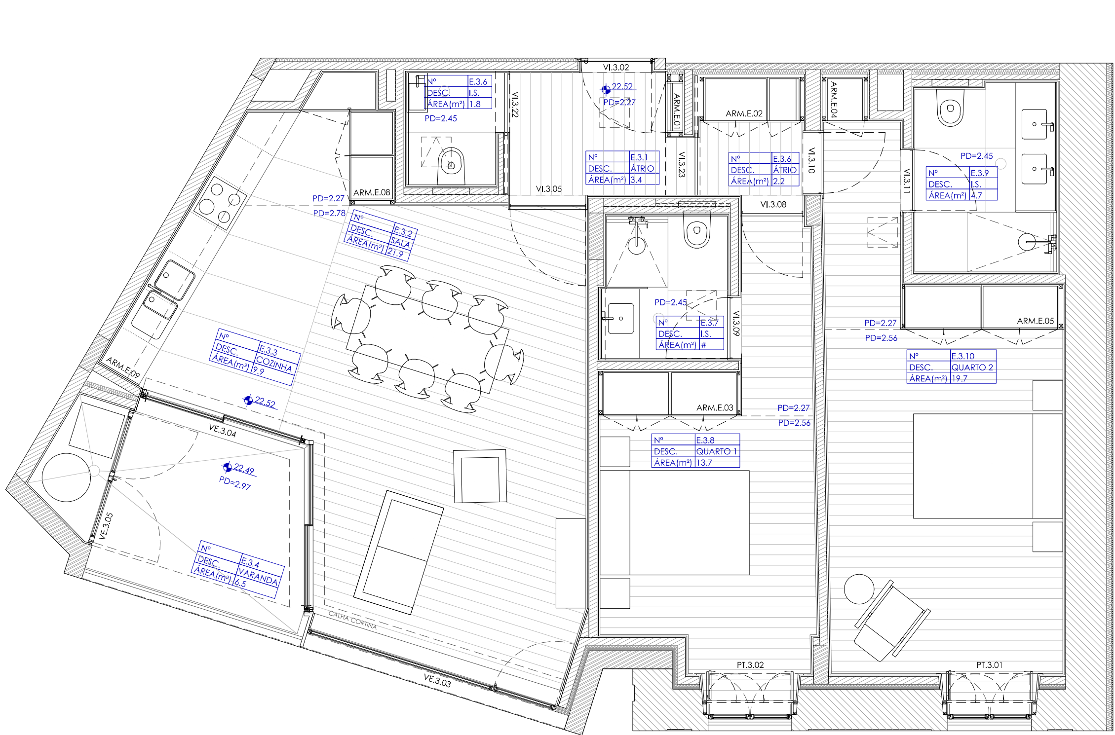
PLANTA FRACÇÃO E TIPOLOGIA T2 A.B.C. 113,75 m²
