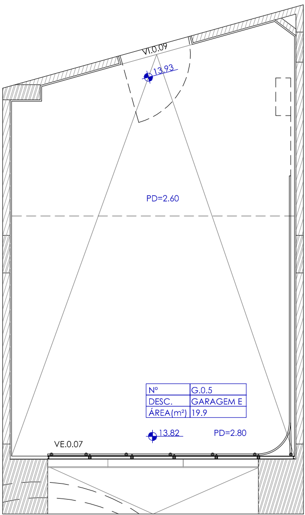
PLANTA GARAGEM FRACÇÃO E A.B.C. 24,85 m²
