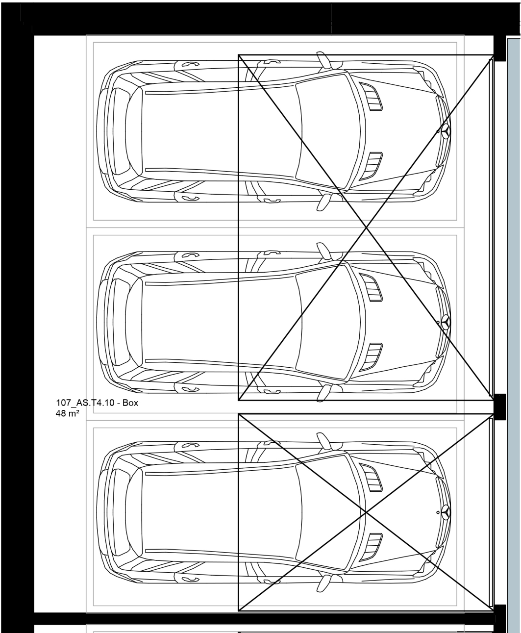
107_AS.T4.10 - Box 1:50
