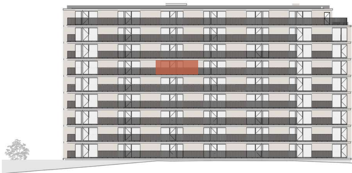
ALÇADO PRINCIPAL
